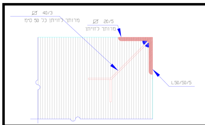
פרט עיגון לזוויתן בקצה הרמפה
